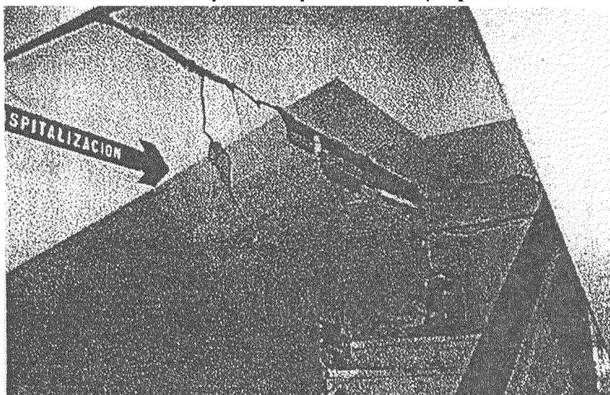
Foto 12. Daños en paredes de escaleras (Hosp. Miguel Alcívar)
