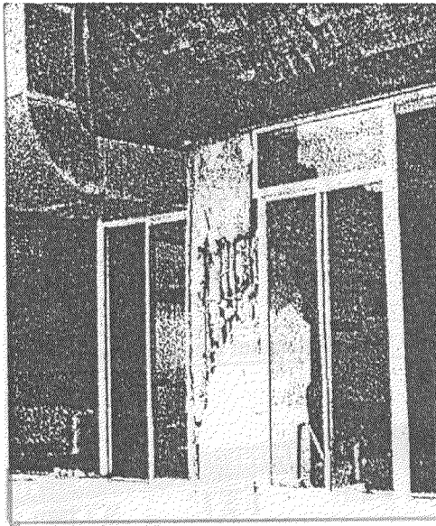
Foto 6. Columna perimetral fallada (Hosp. Miguel Alcívar)
