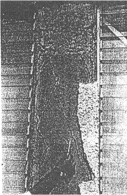
Foto 4. Agrietamiento en una de las columnas Perimetrales (Hosp Miguel Alcívar)
