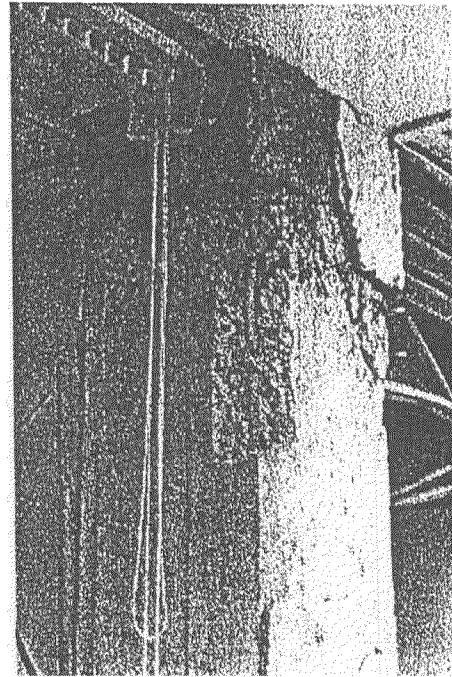
Foto 5. Desconchamiento en otra columna perimetral (Hosp. Miguel Alcívar)
