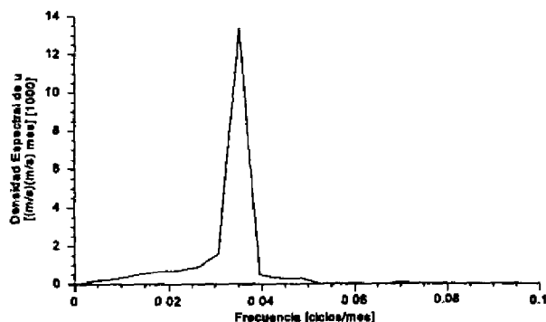
Fig. 6 Densidad espectral de la anomalía suavizada del viento zonal (u) en 50 hPa, estación Juan Santamaría, 1972-92.
