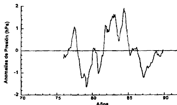
Fig. 2. Anomalías de la diferencia de presión media mensual entre Limón y Liberia, 1976-90.
