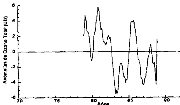
Fig. 7. Anomalías de ozono total sobre Costa Rica, 1978-88.
