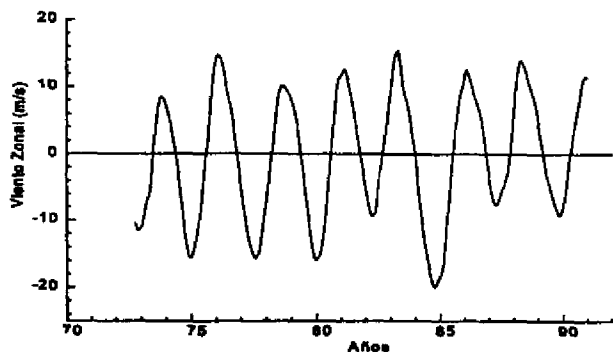
Fig. 5. Oscilación Cuasi-Bienal (OCB) en 50 hPa, 1972-92
