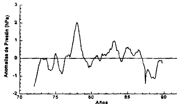
Fig. 1. Anomalías de la diferencia de presión media mensual entre Limón y Puntarenas, 1972-90.
