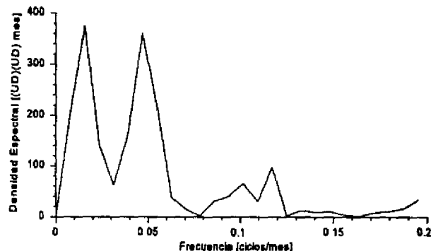
Fig. 8. Densidad espectral de la anomalía del ozono total, 1978-88.
